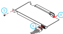
图2-10 显卡安装
