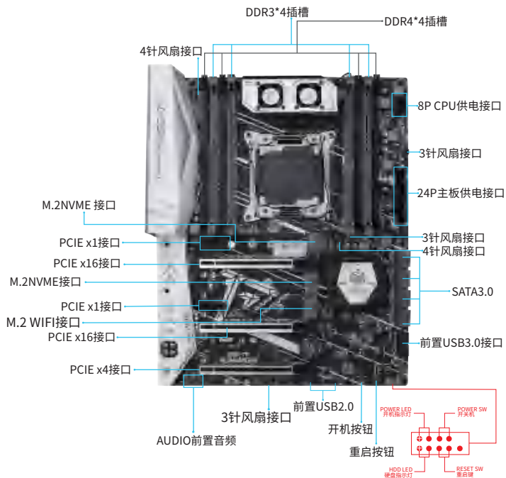
图1-1 X99-TF 主板图解
